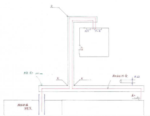
【電線工事掘削図】
